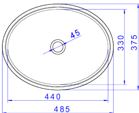
Desenho Técnico
